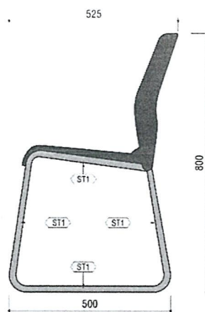
MẶT HÔNG
