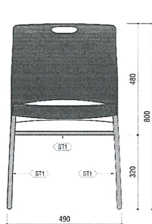
MẶT TRƯỚC
